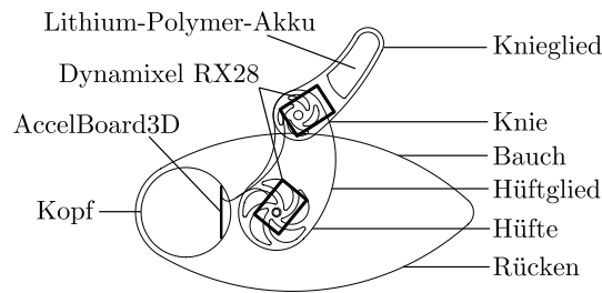
Abbildung 29: Abgebildet ist eine schematische Darstellung des Semni. Wichtige Komponenten wie das Controller-Board, Motoren und Akku sind extra ausgewiesen. Außerdem sind nochmal die Bezeichnungen der Körperteile aufgeführt.
