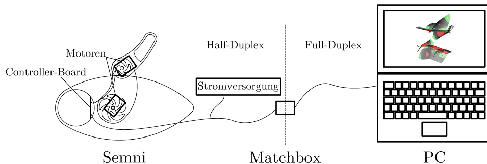
Abbildung 28: Gezeigt ist der schematische Aufbau für das ABC-Learning. Ein PC ist über USB mit einer sogenannten Matchbox verbunden, welche den Semni und PC galvanisch entkoppelt und USB zu RS-485 konvertiert. Der Semni ist über RS-485 ebenfalls mit der Matchbox verbunden. Auf diesem Weg können der Semni und PC miteinander kommunizieren.
