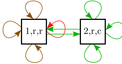
Abbildung 55: Abgebildet ist ein einfaches Beispiel eines sensomotorischen Graphen mit verschiedenen Situationen. Zu sehen sind zwei Postures und verschiedene Verbindungen. Rote und grüne Übergänge gehören jeweils zu verschiedenen Situationen, während braune Übergänge zu beiden Situationen gehören.
