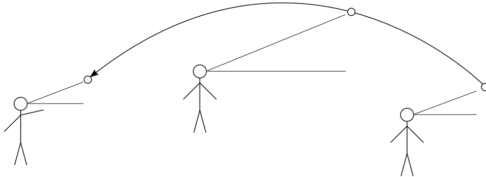
Abbildung 13: Indem der Spieler den Blickwinkel zum Ball konstant hält, schafft er es den Aufschlagorts des Balls zu erreichen und ihn dort fangen zu können. Dies wird als die „Gaze“-Heuristik in McLeod u. Dienes (1996) bezeichnet.
