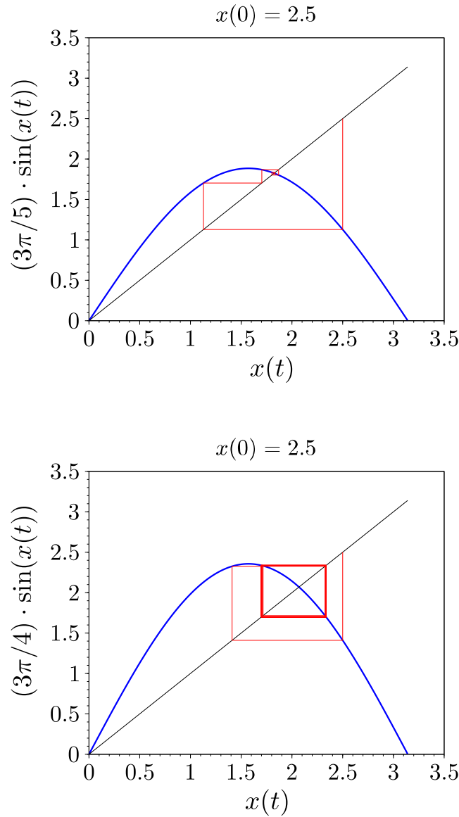
Abbildung 9: Dargestellt sind hier zwei Cobweb-Diagramme des dynamischen Systems mit der Übergangsfunktion x(t) = (a\pi/2) \cdot \sin(x(t-1)) mit verschiedenen Werten für a . Oben ist zu sehen, dass es einen stabilen Fixpunkt gibt, dieser jedoch im Vergleich zu Abbildung 8 verschoben ist. Es handelt sich hierbei nicht um eine Bifurkation. Im unteren Diagramm ist zu sehen, dass ein 2-periodischer Orbit entstanden ist. In diesem Fall liegt eine Bifurkation vor.
