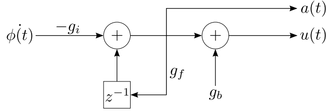
Abbildung 16: Abgebildet ist eine kompaktere Darstellung des CSL. Anstatt eines Winkels bildet die Winkelgeschwindigkeit den sensorischen Eingang. Zusätzlich wurde für die weitere Erklärung eine Zwischenvariable a(t) eingefügt.
