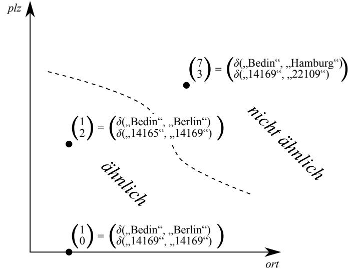
Abbildung 4.2.: Abbildung von Datensatzpaaren auf Vektoren
