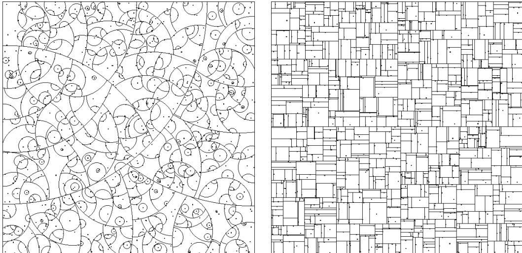
Abbildung 3.1.: Kugel-Partitionierung und Hyperebenen-Partitionierung [Yia93]
