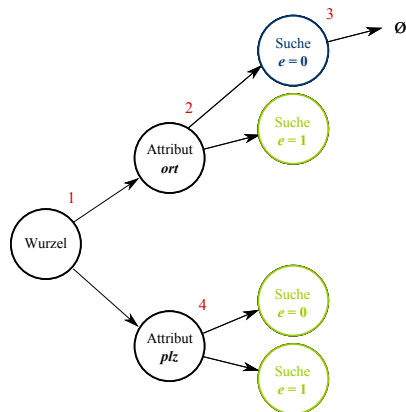
Abbildung 5.7.: Beispiel (Schritte 1–4)
