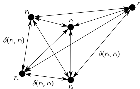
Abbildung 2.1.: Metrischer Raum
