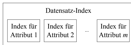
Abbildung 5.1.: Indexstrukturen-Architektur
