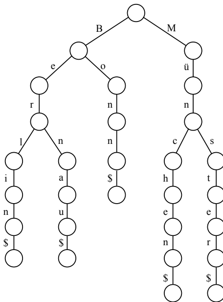
Abbildung 5.2.: Trie mit fünf Zeichenketten
