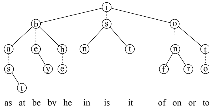
Abbildung 5.4.: Ternary Search Trie mit 12 zwei-buchstabigen Wörtern [BS97]
