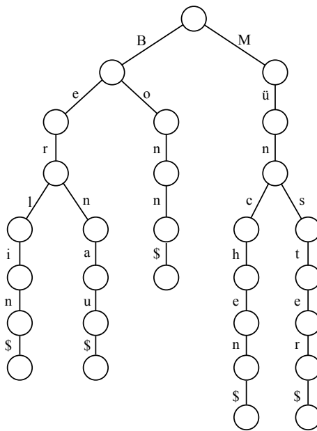
Abbildung 3.2.: Trie mit fünf Zeichenketten
