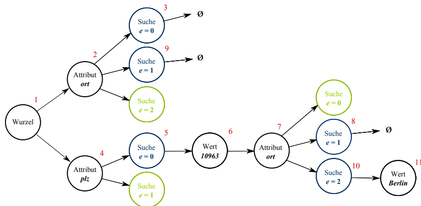
Abbildung 5.9.: Beispiel (Schritte 9–11)
