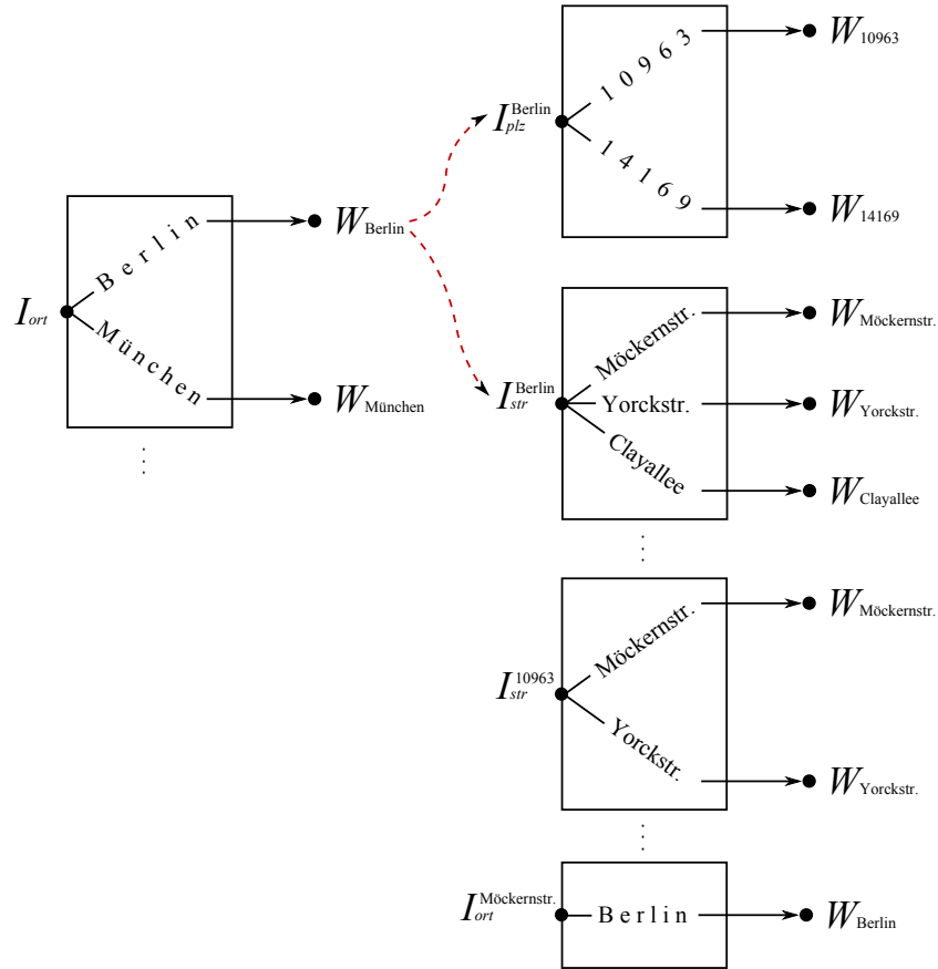
Abbildung 5.5.: Datenstruktur beim FRI (Ausschnitt des Beispiels)
