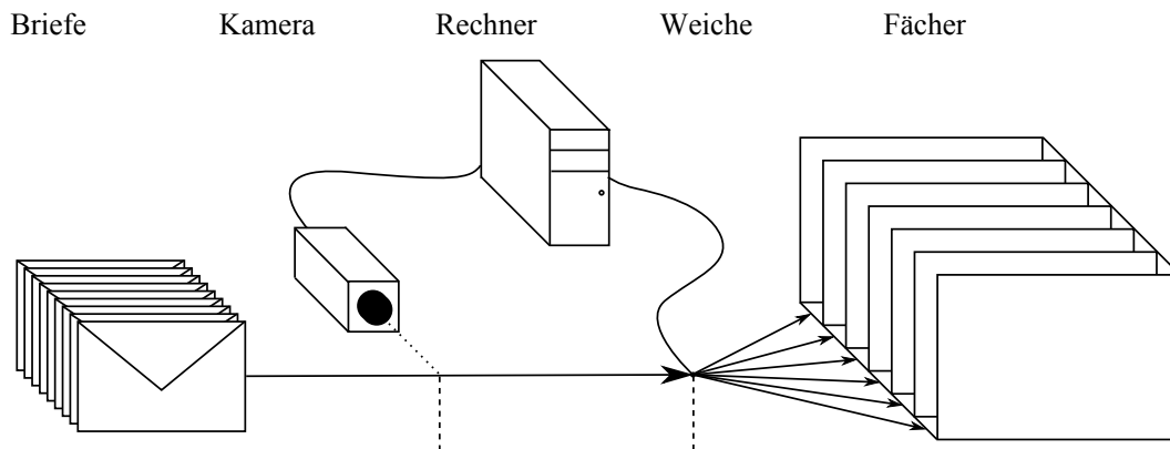
Abbildung 1.2.: Briefsortiermaschine (schematisch)
