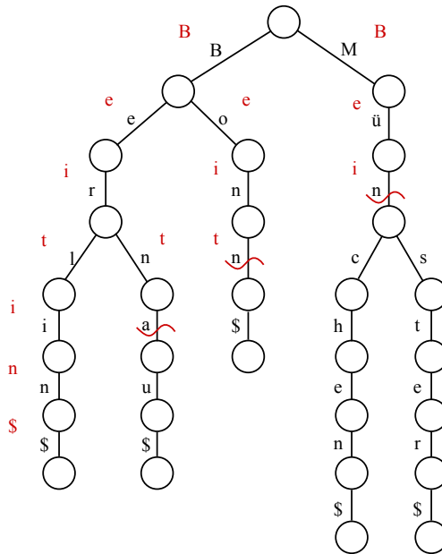
Abbildung 5.3.: Ähnlichkeitssuche in einem Trie mit q = \text{„Beitin“} und e = 2
