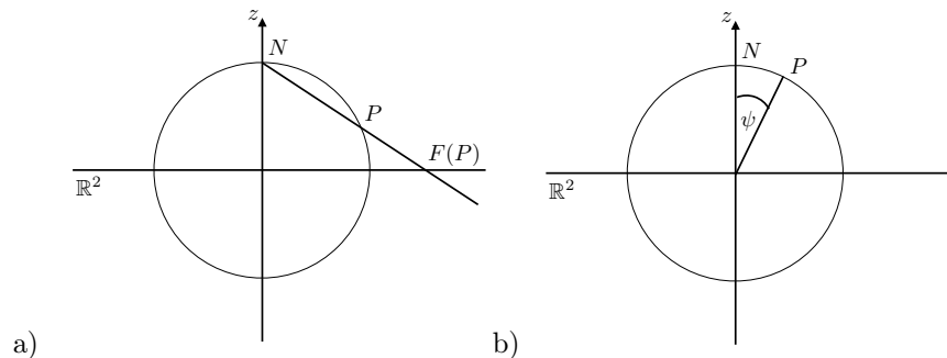
Figure 1: Stereographische Projektion und Definition des Polarwinkels \psi .
